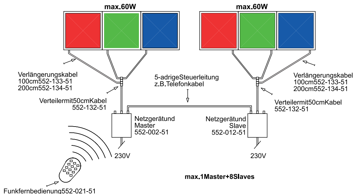
Leuchtkästen 552-550-98/552-551-98
