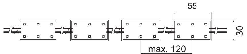
21x6 SMD-Dioden(0,5W/Modul)
